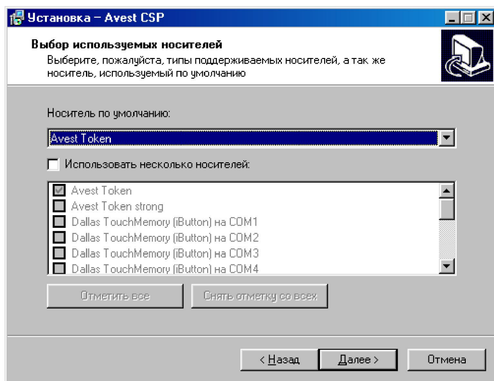
Рисунок 4 - Выбор носителя личных ключей по умолчанию.
